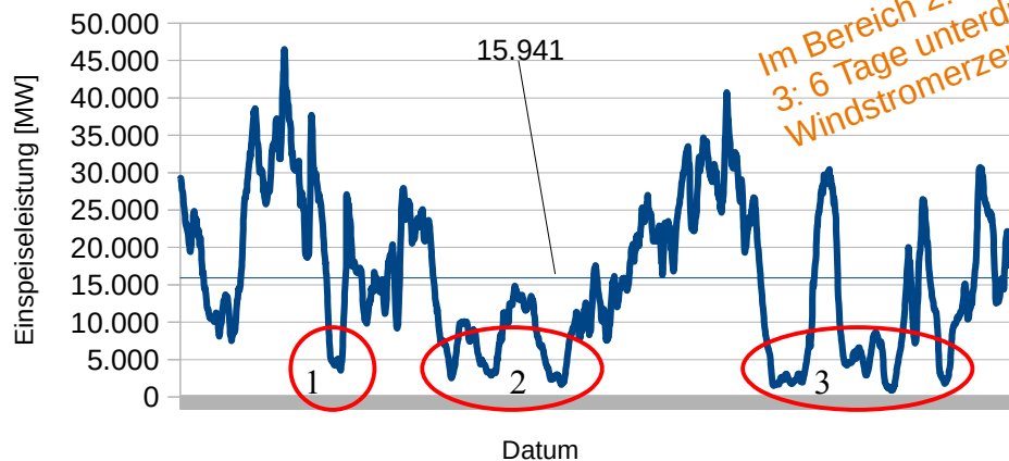
Windstromeinspeisung September 2026
