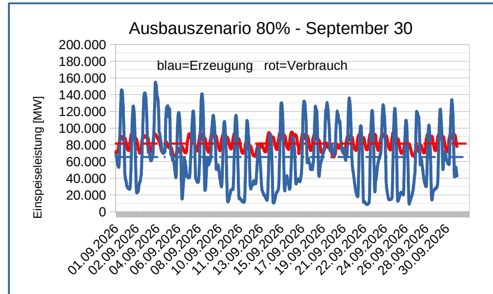
Diagramm 2: Verläufe von Ökostromerzeugung (Wind, PV, Biomasse und Wasserkraft), hochgerechnet aus September 2026 entspr. Planungsziel BMWK für September 2030
