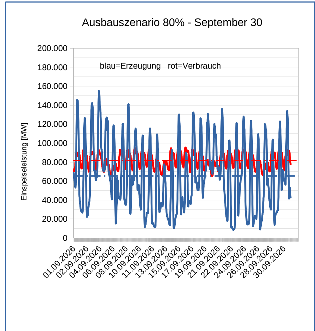
Diagramm 2: Verläufe von Ökostromerzeugung (Wind, PV, Biomasse und Wasserkraft), hochgerechnet aus September 2026 entspr. Planungsziel BMWK für September 2030
