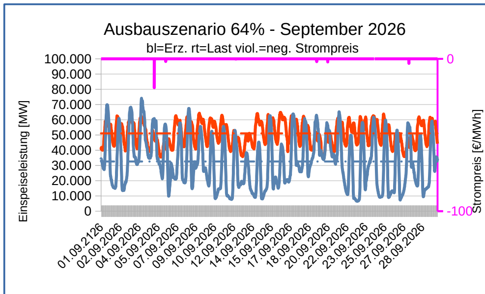
Diagramm 1: Verläufe von Ökostromerzeugung (Wind, PV, Biomasse und Wasserkraft) und Stromverbrauch bei aktuellem Ausbaustatus September 2026.
