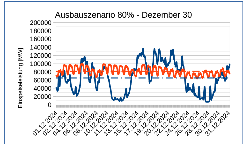
Diagramm 2: Verläufe von Ökostromerzeugung (Wind, PV, Biomasse und Wasserkraft), hochgerechnet aus Dezember 2024 entspr. Planungsziel BMWK für Dezember 2030
