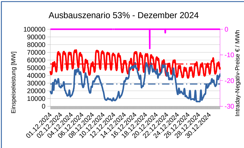
Diagramm 1: Verläufe von Ökostromerzeugung (Wind, PV, Biomasse und Wasserkraft) und Stromverbrauch bei aktuellem Ausbaustatus Dezember 2024
