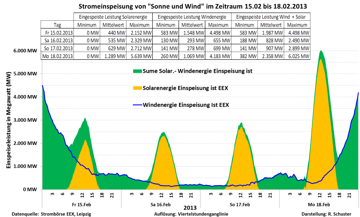
Diagramm 6: Lastganglinie (Einspeiseleistung pro Zeit) aller deutschen Windenergie- und Fotovoltaik-Anlagen mit aktuell 62 000 MW Nennleistung im Februar 2013
