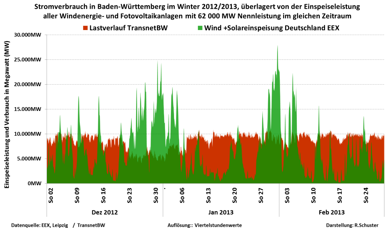
Diagramm 7: Einspeiseleistung aller Windenergie- und Fotovoltaik-Anlagen in Deutschland relativ zur Stromverbrauchskurve für Baden-Württemberg (Band bis ca. 10 000 MW) im Winter 2013
